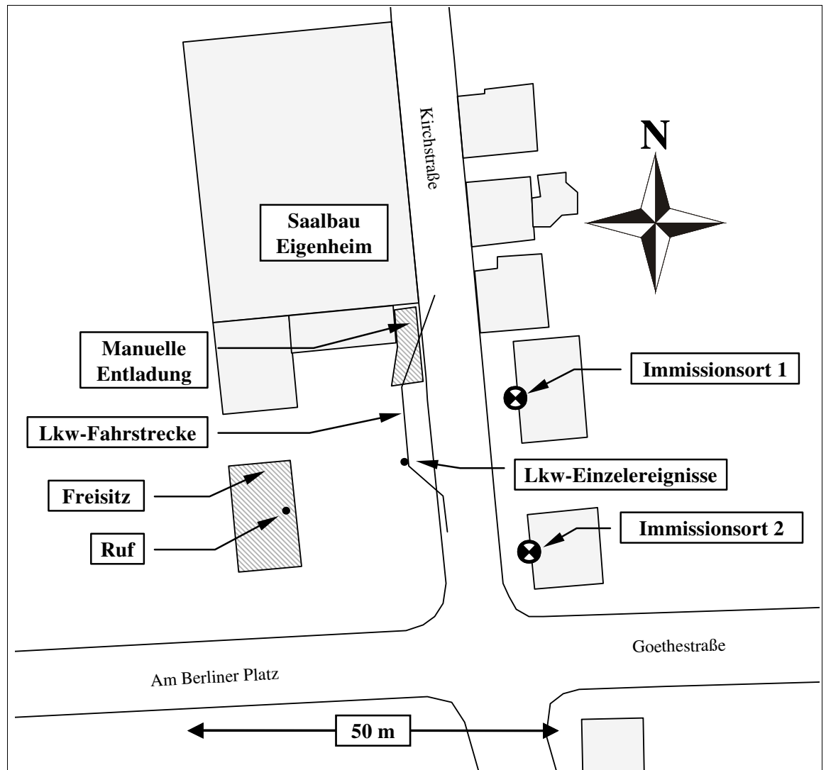
Abb. 2 : Übersichtsplan der Umgebung mit Kennzeichnung der Immissionsorte und Schallquellen (Fall A).
