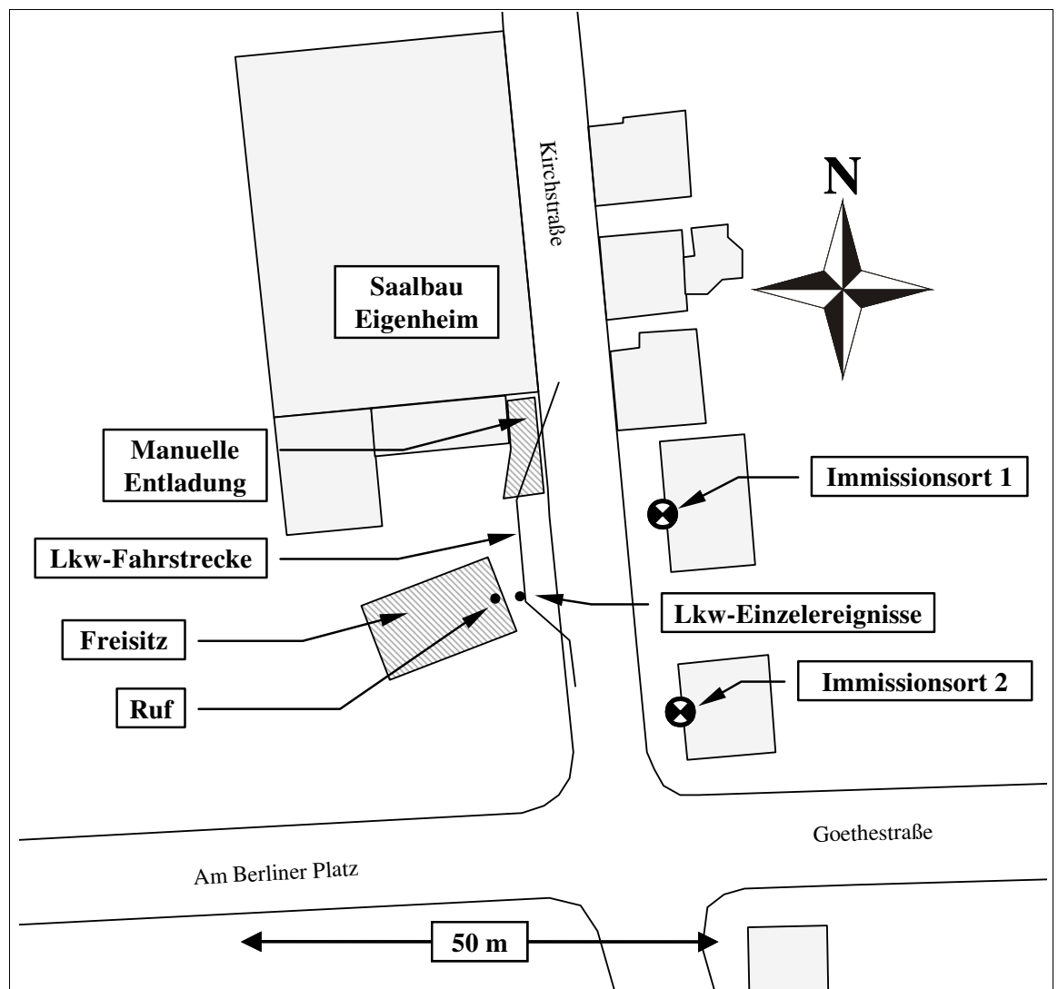
Abb. 3 : Übersichtskarte der Umgebung mit Kennzeichnung der Immissionsorte und Schallquellen (Fall B).
