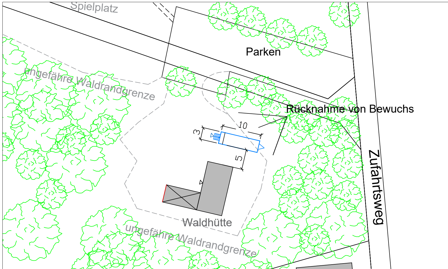
Grundriss und Ansicht Waldkindergarten
