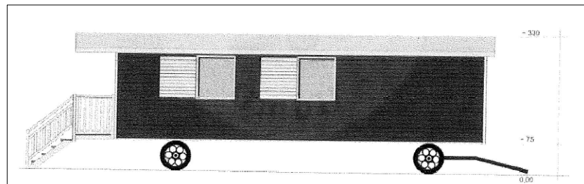
Grundriss und Ansicht Waldkindergarten
