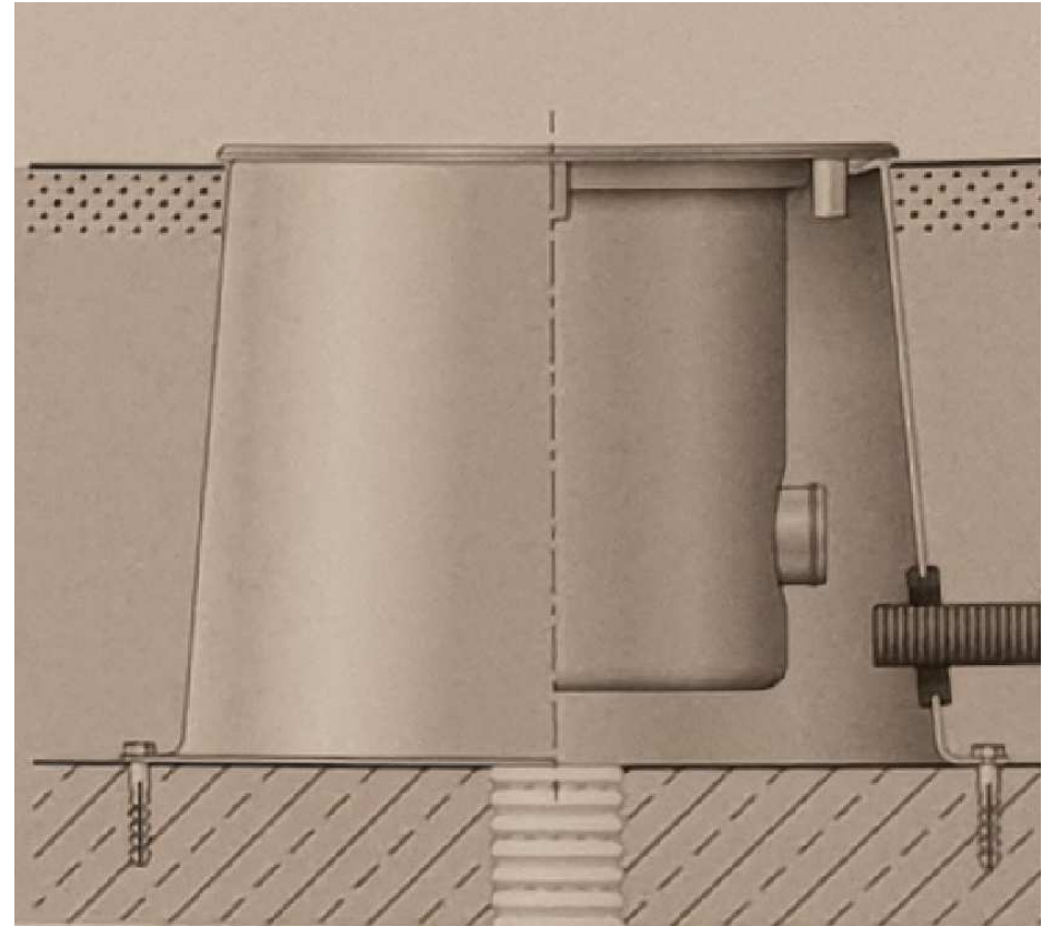
Fundament muss bauseits hergestellt werden
