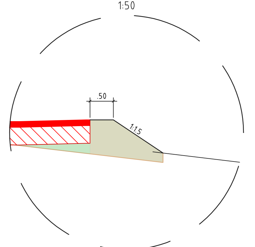
BÖSCHUNG - DAMM
