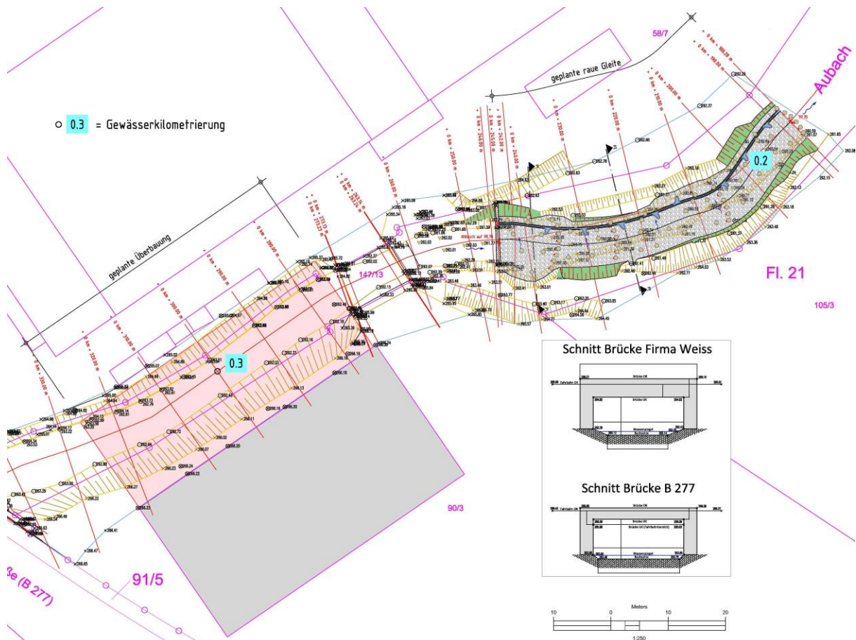
Abb. 2: Lageplan der Fachplanung mit Darstellung der Rauhen Gleite und dem geplanten überbauten Bereich des Aubaches, Quelle: Wasserrechtliches Genehmigungsverfahren 2021, erstellt Büro Falkenhahn, Fulda
