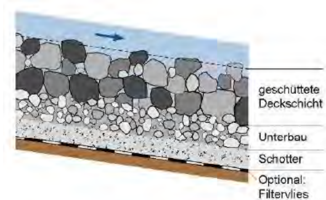
Bild 236: Aufbau eines geschütteten Raugerinnes (Grafik: DUMONT)
