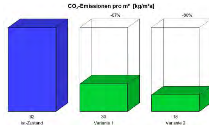
Abbildung 37: Vergleich der CO 2 -Emissionen der Varianten
