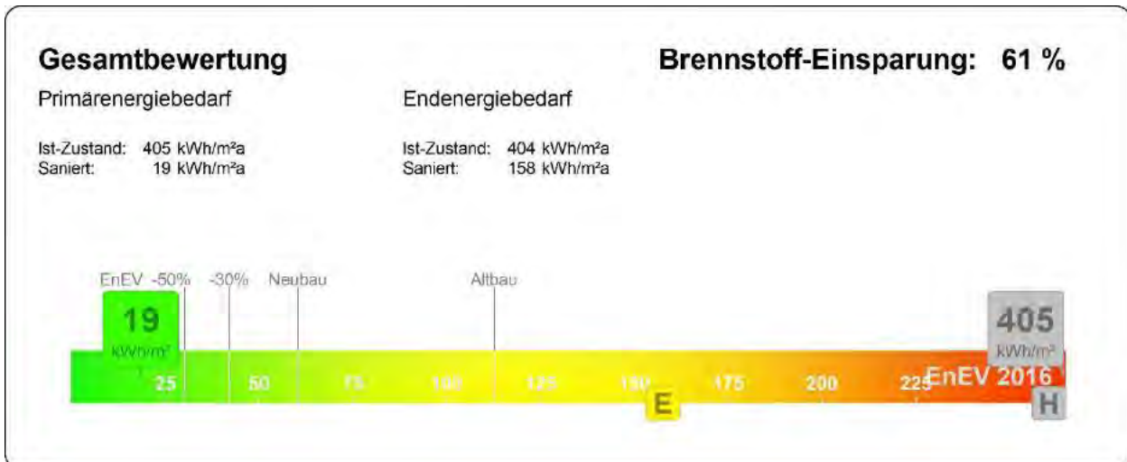
Abbildung 39: EnEV-Gesamtbewertung – Variante 2
