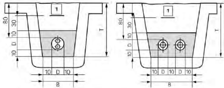
Abbildung 42: Einbausituation für die Nahwärmeleitungen
