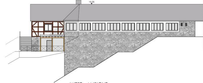
WEST - ANSICHT
