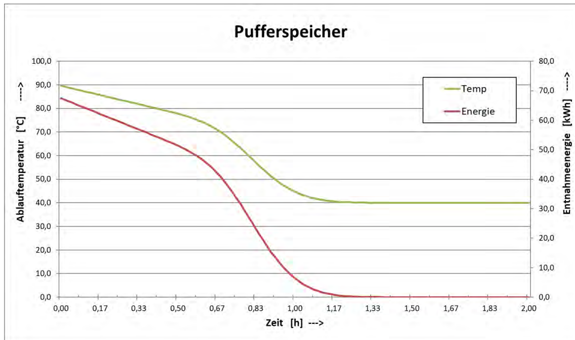
Abbildung 45: Entnahmeganglinie für die beiden Pufferspeicher.
