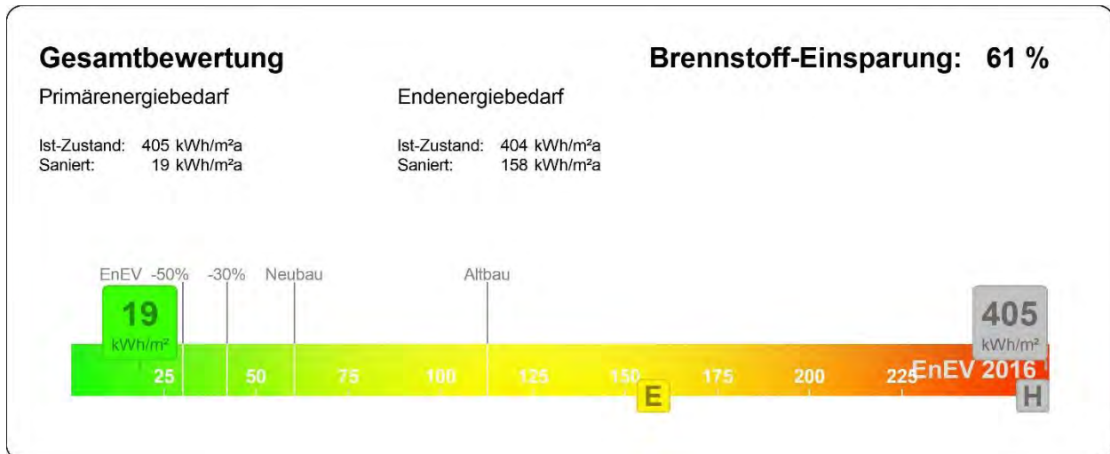
Abbildung 39: EnEV-Gesamtbewertung – Variante 2
