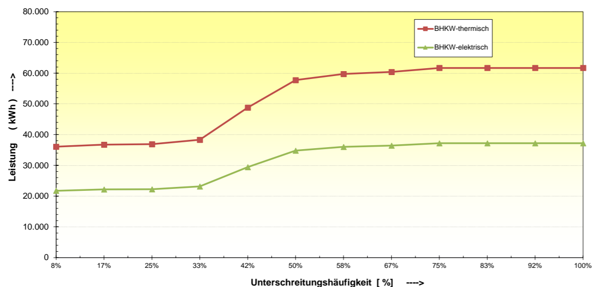
Nahwärmenetz - Dauerlinie für den Betrieb vom BHKW -
