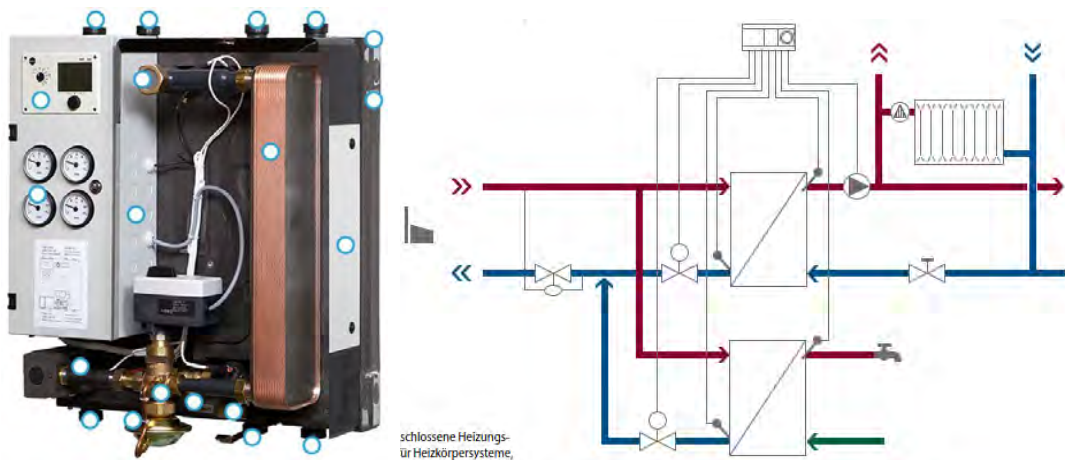
Abbildung 43: Beispiel für eine Hausübergabestation
