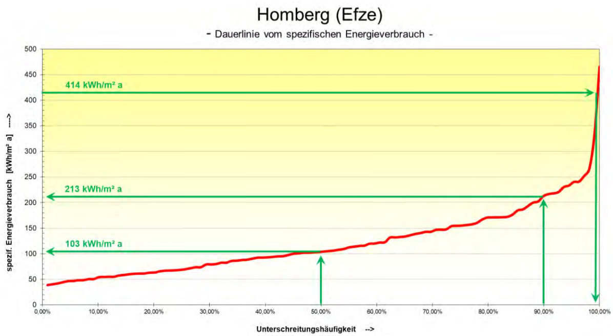
Abbildung 34: Dauerlinie des jährlichen spezifischen Energieverbrauchs
