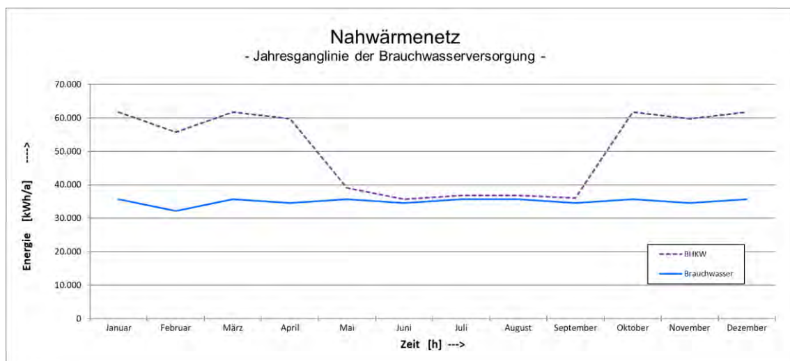
Abbildung 44: Ganglinie der Grundlast und Grundlastversorgung
