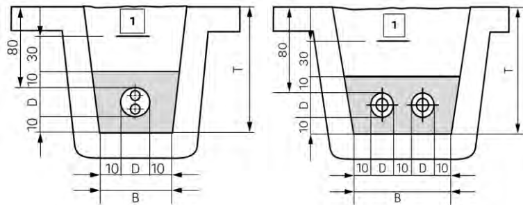
Abbildung 42: Einbausituation für die Nahwärmeleitungen Quelle: Rehau
