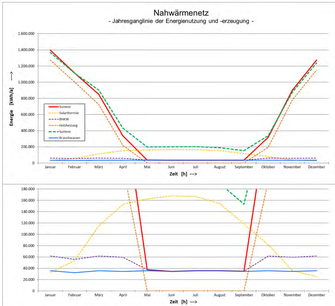
Abbildung 52: Jahresganglinie der Energieerzeugung mit Solarthermie
