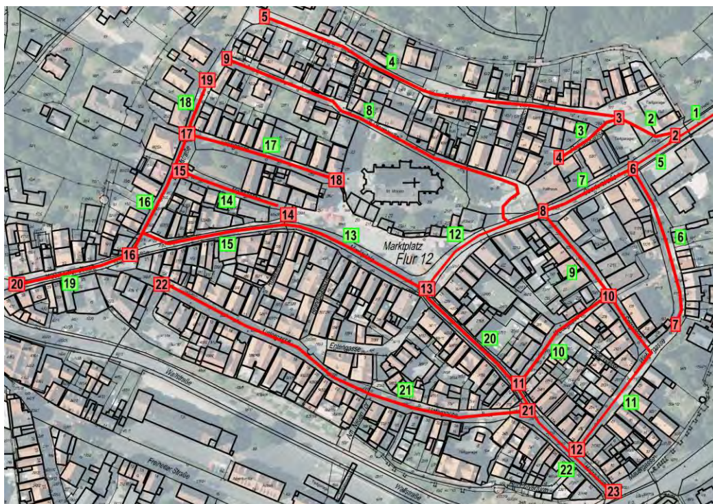
Abbildung 41: Lageplanskizze des Nahwärmenetzes der Altstadt
