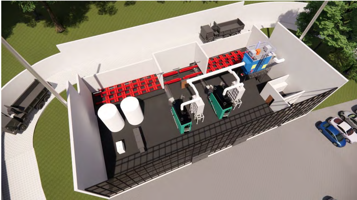
Abbildung 46: Grundriss der Heizzentrale – Innenwände ausgeblendet
