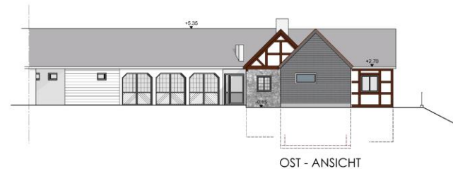
OST - ANSICHT
