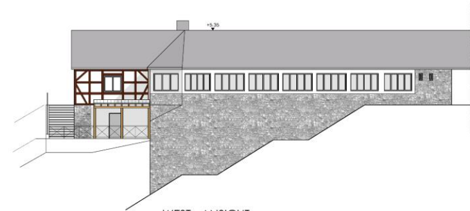
WEST - ANSICHT
