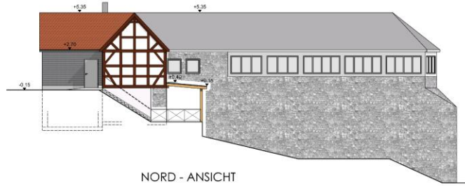
NORD - ANSICHT
