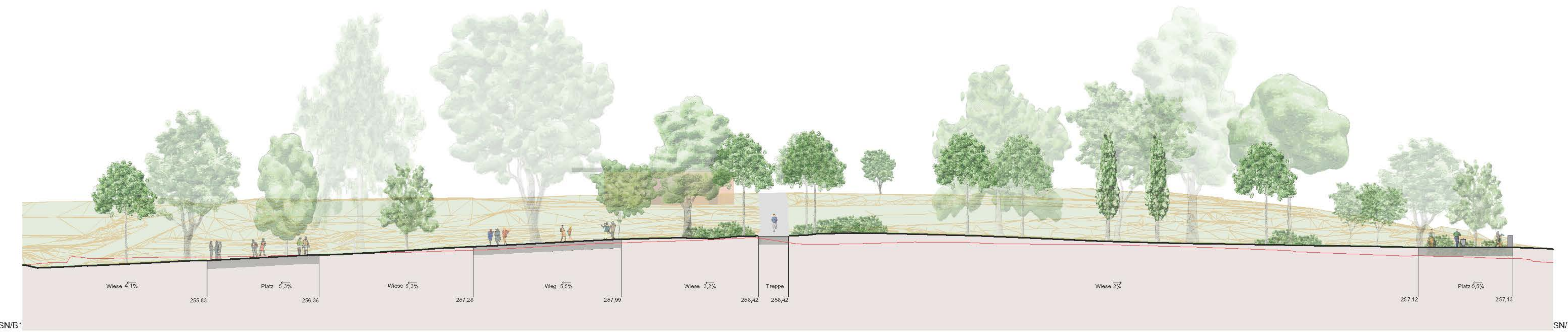
Schnitt B1 1:200
