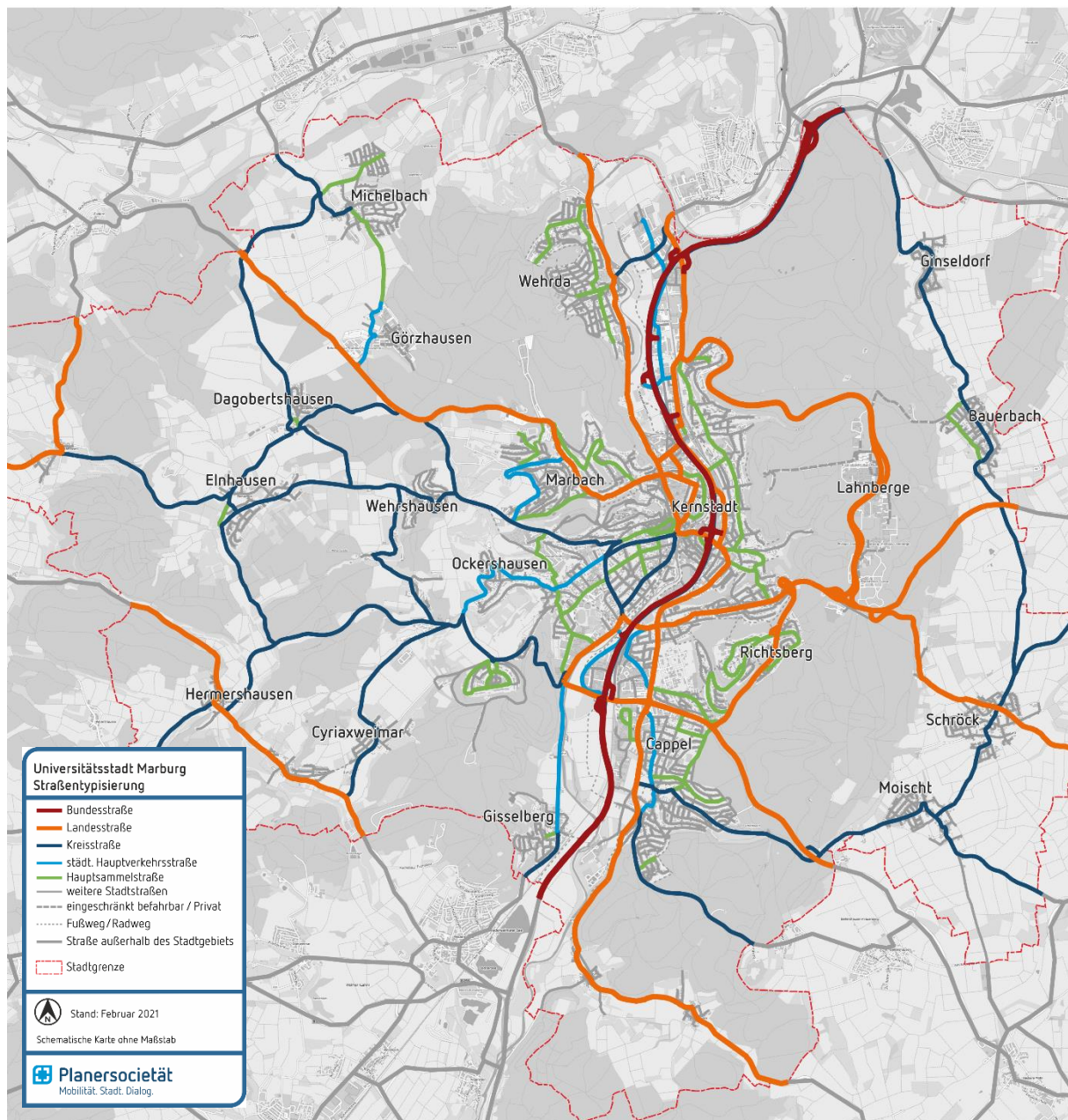
Abbildung 80: Straßennetztypisierung und -klassifikation
