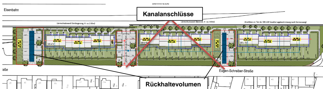
Abb. 13: Entwässerungskonzept
