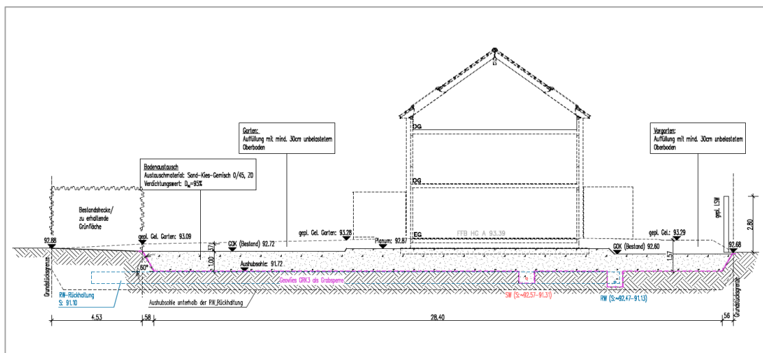
Abb. 7 Geländeschnitt Bodenaustausch Garten HG A
