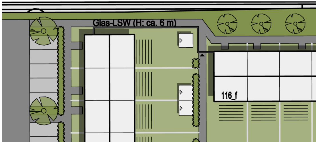
Abb. 16: Lärmschutzwand aus Glas zum Schutz der Gärten | Variante III
