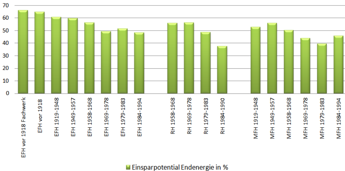
Abb. 51: Energieeinsparpotenziale (Heizung und Warmwasser) der Referenzgebäude
