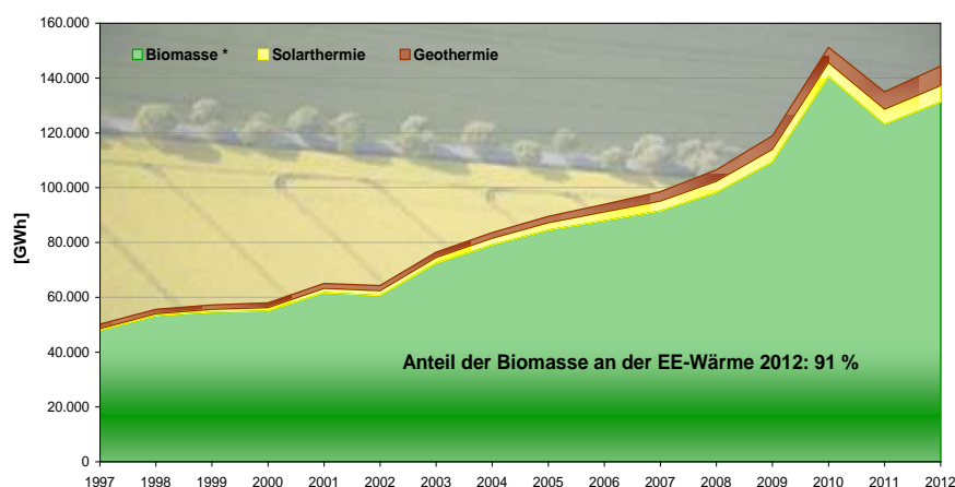
Abb. 41: Bereitstellung der erneuerbarer Energien zur Wärmebereitstellung in den Jahren 1997 bis 2012 der Strombereitstellung aus erneuerbaren Energien in Deutschland 2012 26
