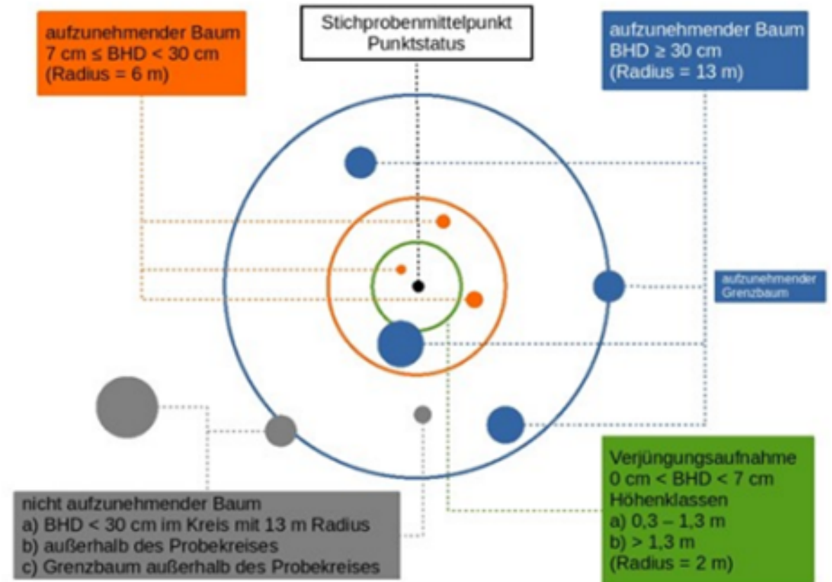
Abbildung 1: Schematische Darstellung Probekreis und Aufnahmebereiche
