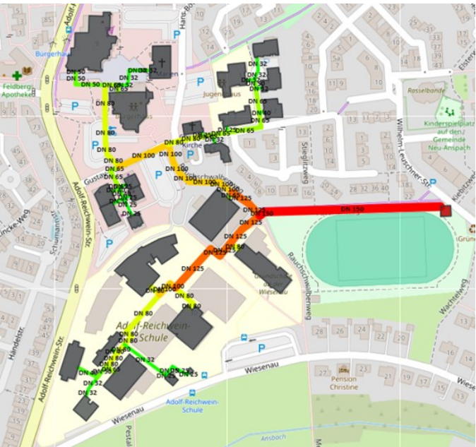
Schematische Darstellung der Gebäude und Trassenführung
