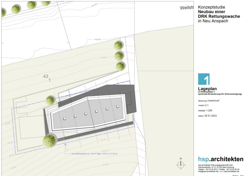
Abb. 3: Freiflächenplan, unmaßstäblich
