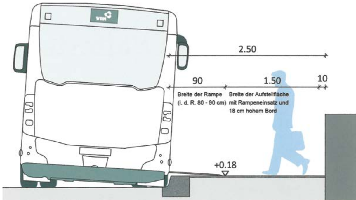
Abb. 12: Einstieg an einem 18 cm Hochbord Breite der Aufstellfläche 2,50 m (ca. 1 m Rampe + 1,50 m Rangierfläche für Rollstuhlnutzende), Rampeneinsatz erforderlich, Überstreichbarkeit möglich
