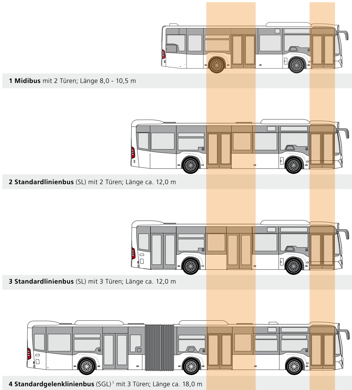
Abb. 9: Türpositionen der unterschiedlichen Bustypen
