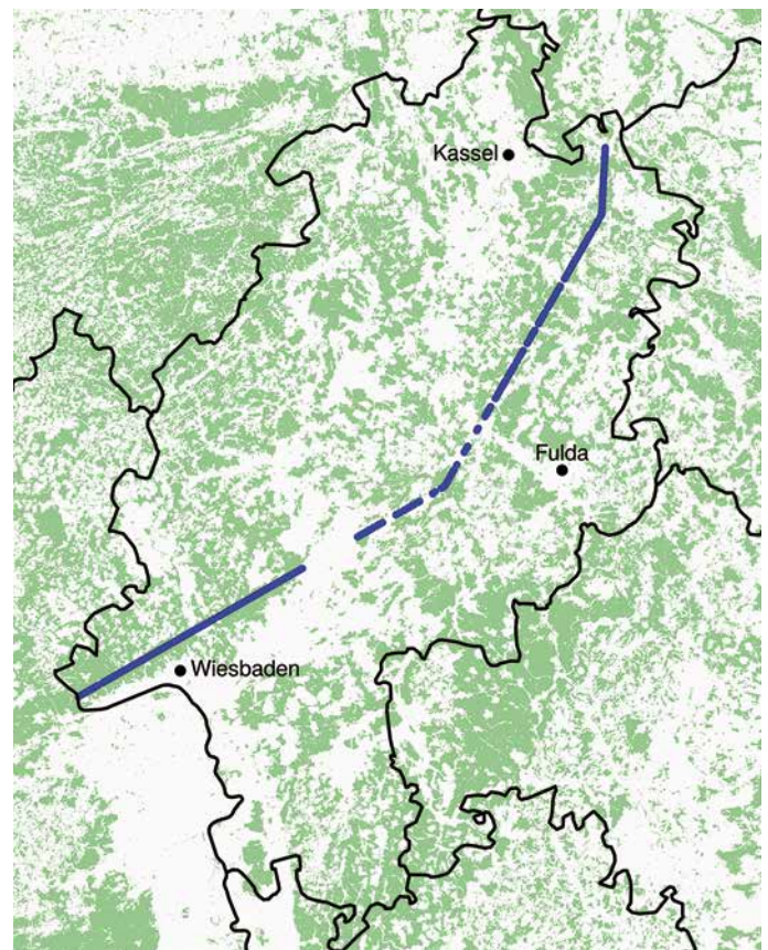
Transekt von Witzzenhausen (Werra) über den Meißner, den Vogelsberg, die Wetterau und den Hohen Taunus bis zum Rhein bei Rüdesheim. Für diesen Transekt wird die Wuchsleistung für die Jahre 2000 und 2100 projiziert. Der Transekt beinhaltet ausschließlich Waldflächen.
