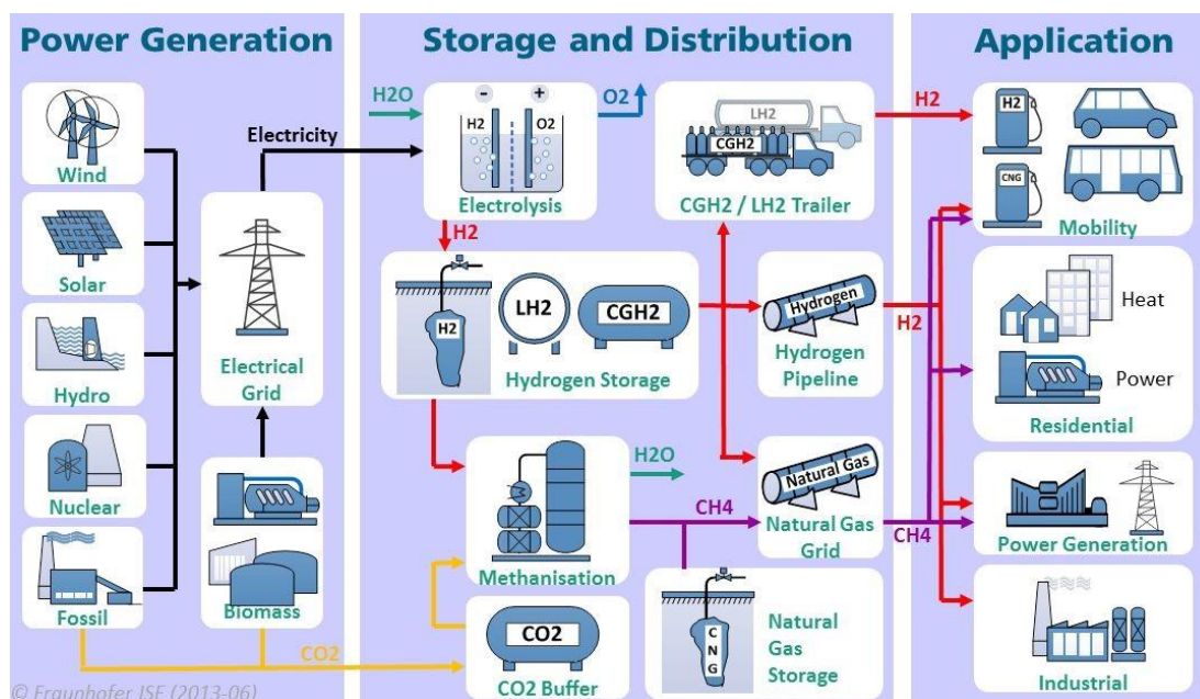
Abbildung 5-16: Allgemeines Funktionsschema des Power-to-Gas-Konzepts (Fraunhofer ISE, 2013)
