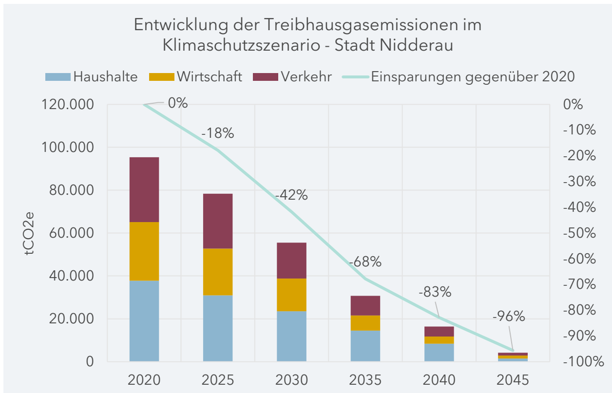
Abbildung 6-11: Entwicklung der Treibhausgasemissionen im Klimaschutzscenario (Eigene Darstellung)
