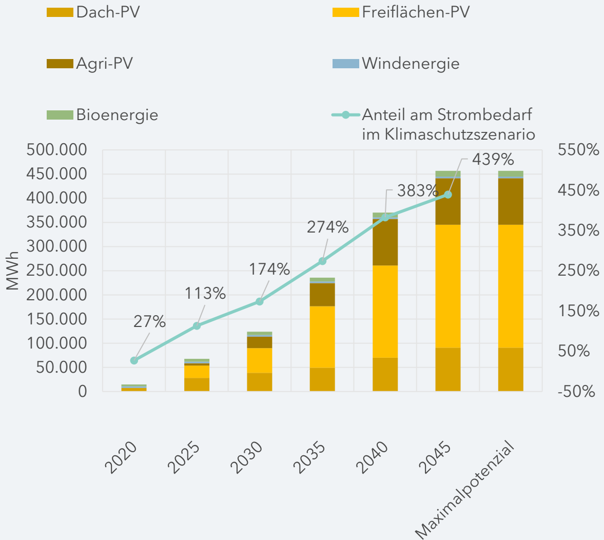
Abbildung 6-6: Kommunenspezifischer Ausbaupfad der Erneuerbaren Energien und Gegenüberstellung des Maximalpotenzials bis zum Zieljahr 2045 (Eigene Darstellung)
