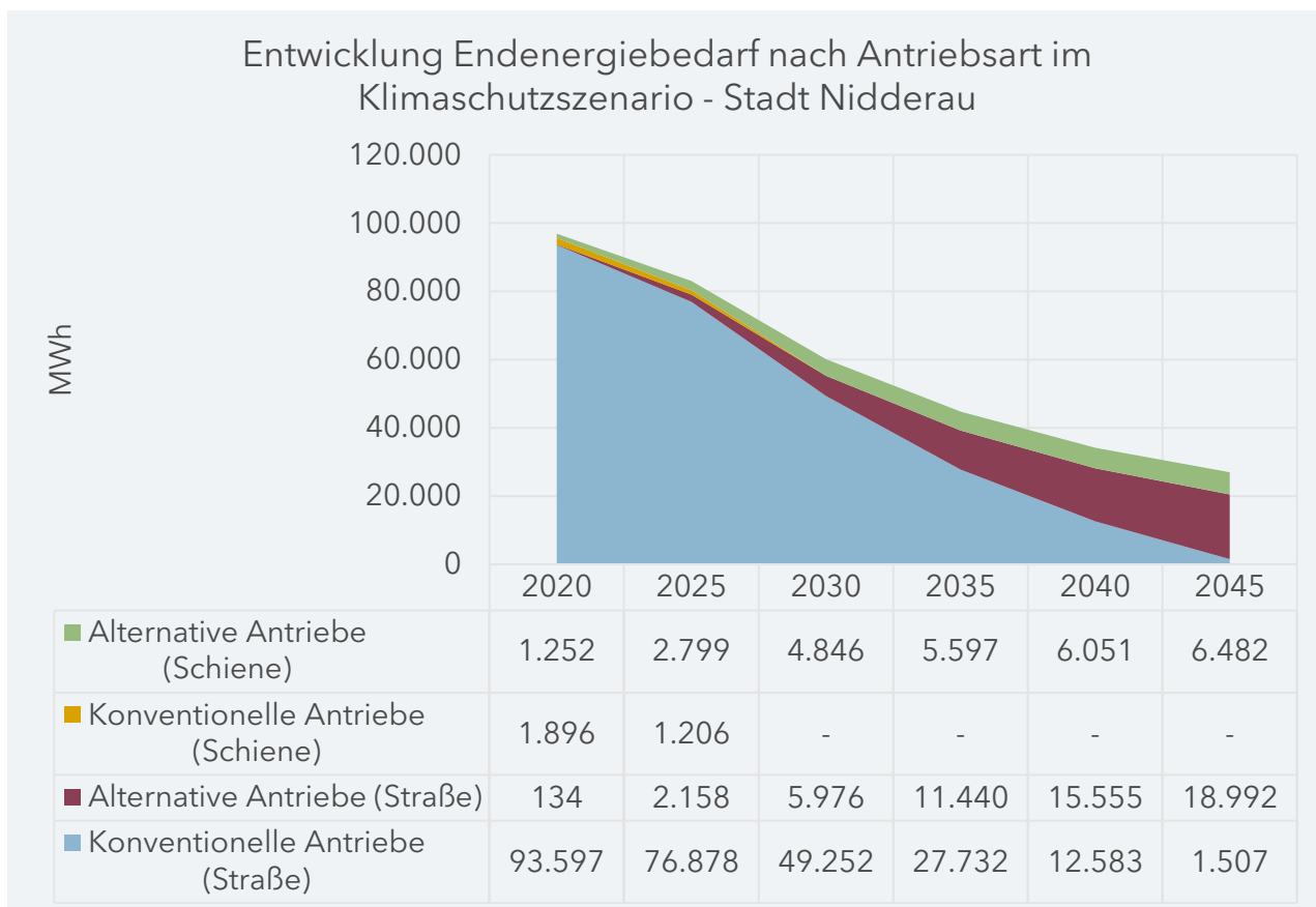
Abbildung 6-4: Entwicklung Endenergiebedarf im Klimaschutzscenario (eigene Darstellung)
