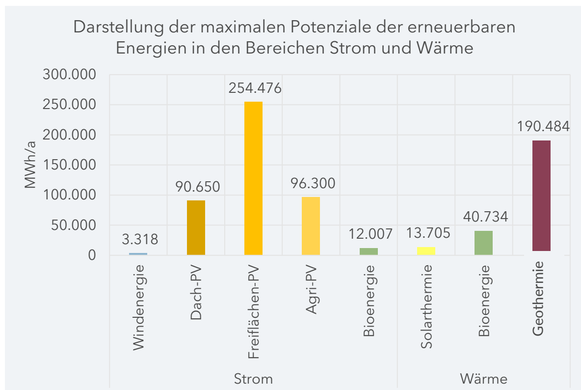
Abbildung 5-15: Darstellung der Maximalen Potenziale der erneuerbaren Energien in den Bereichen Strom und Wärme (eigene Darstellung)
