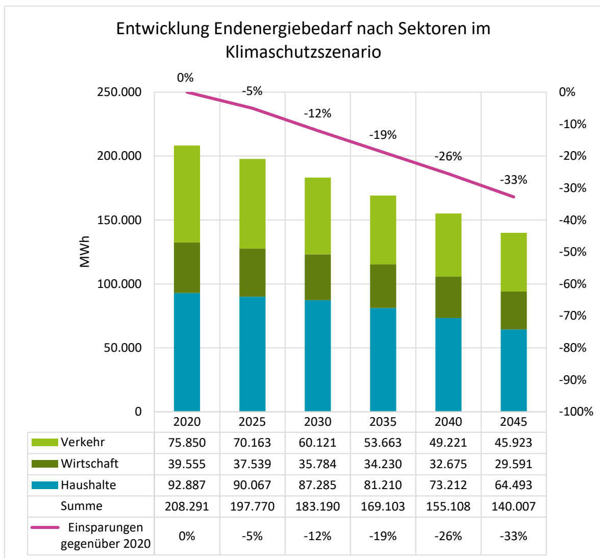
Abbildung 58: Entwicklung des Endenergieverbrauchs nach Sektoren im Klimaschutzszenario
