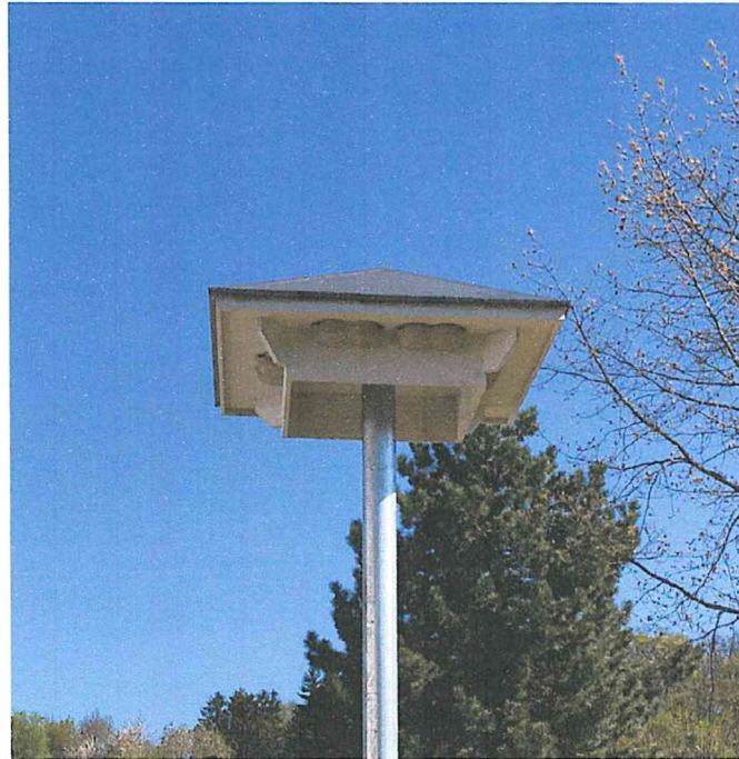
Grundmaße ca. 1,60 x 1,60 x 0,65 m, verzinkte Rohrsäule als Kippmast mit U-Profilen, Gesamthöhe ca. 5,50 m
