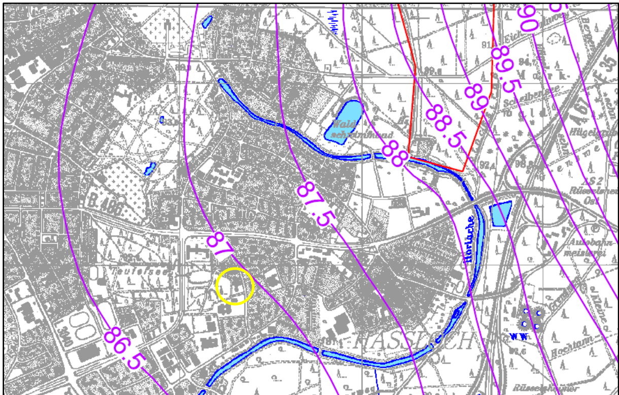
Abbildung 4: Grundwassergleichen April 2001 (Gutachten „Bemessungsgrundwasserstände in Rüsselsheim“, BGS, Darmstadt v. 2006)
