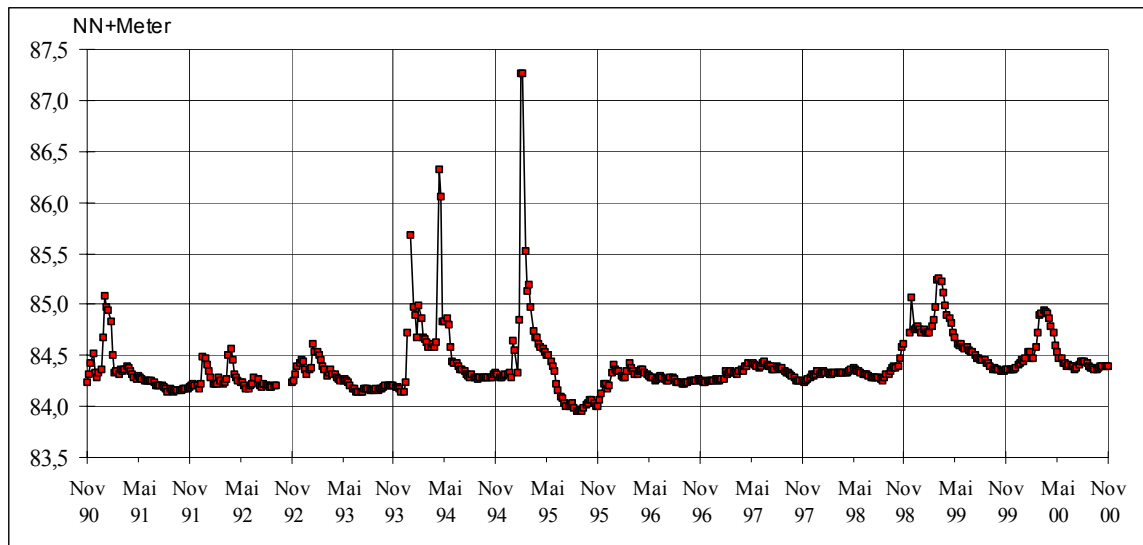
Abbildung 6 Grundwasserstandsganglinie Messstelle 507150 (1990 - 2000)
