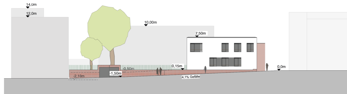
Ansicht Süd
