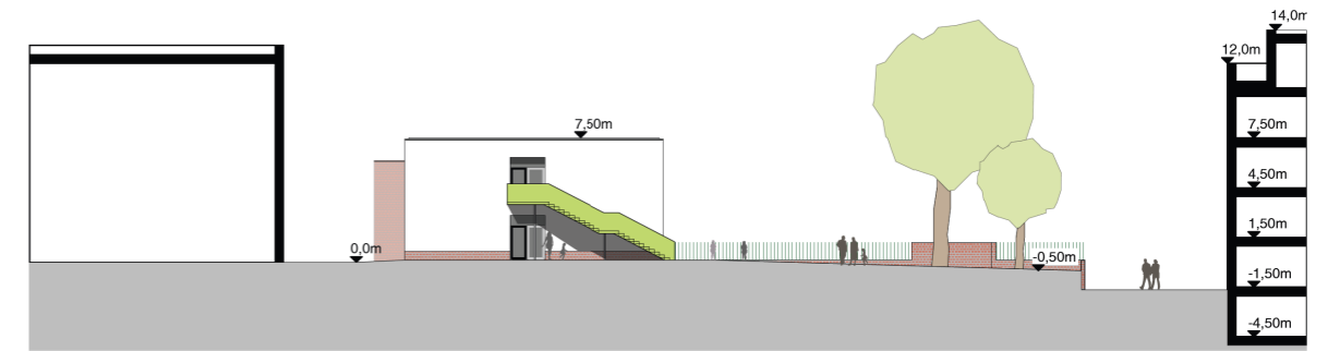
Ansicht Nord
