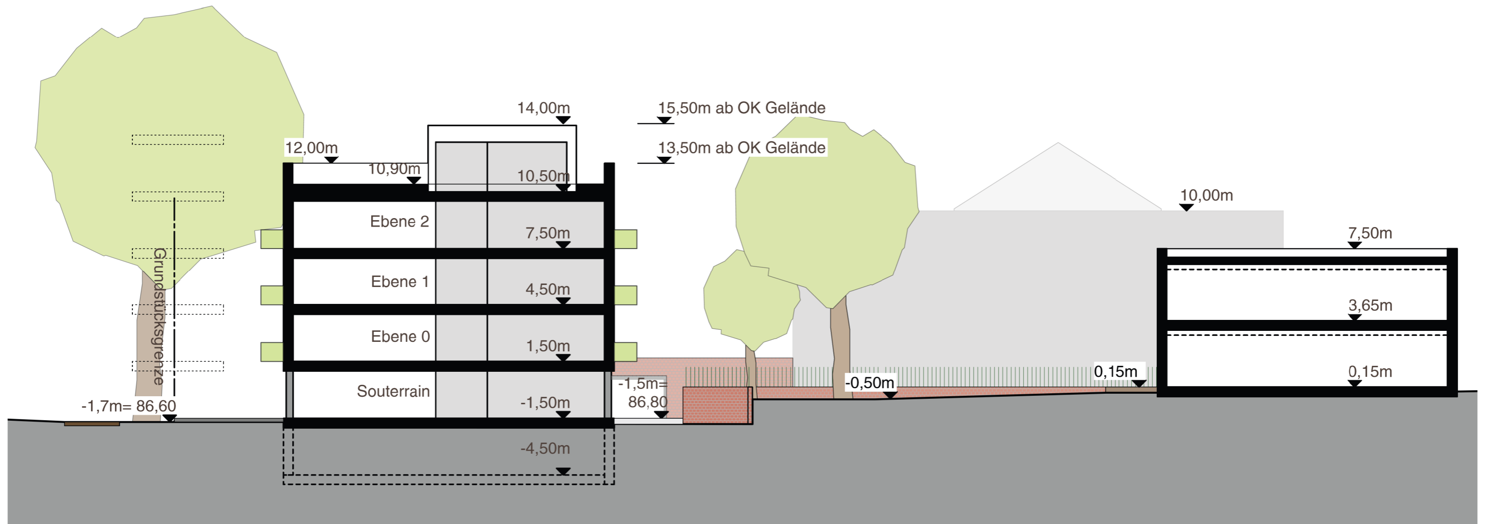
Schnitt B 1:200
