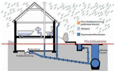
mit Rückstauklappe
