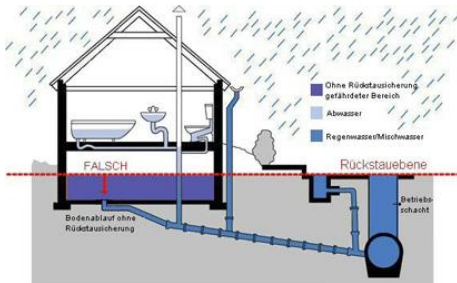
ohne Rückstausicherung
