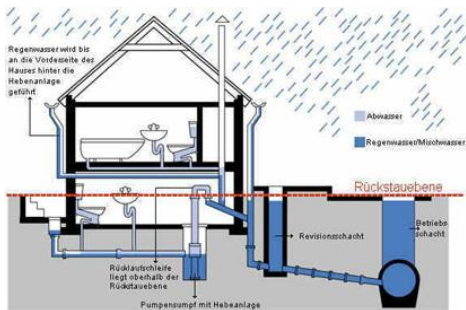
mit Hebeanlage
