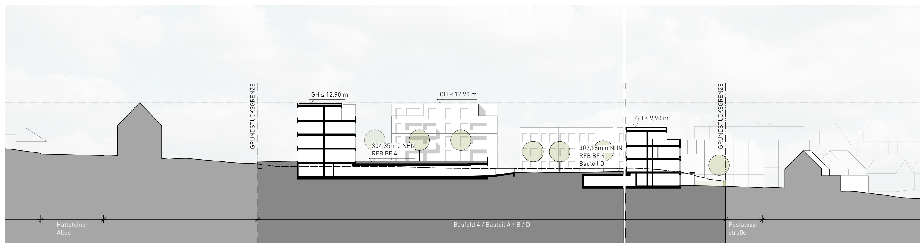
Schnitt C-C
