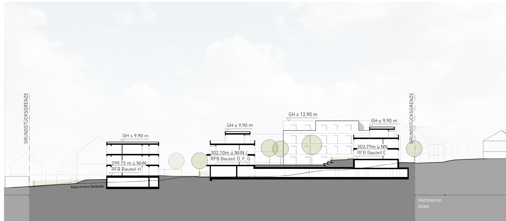
Schnitt A-A
