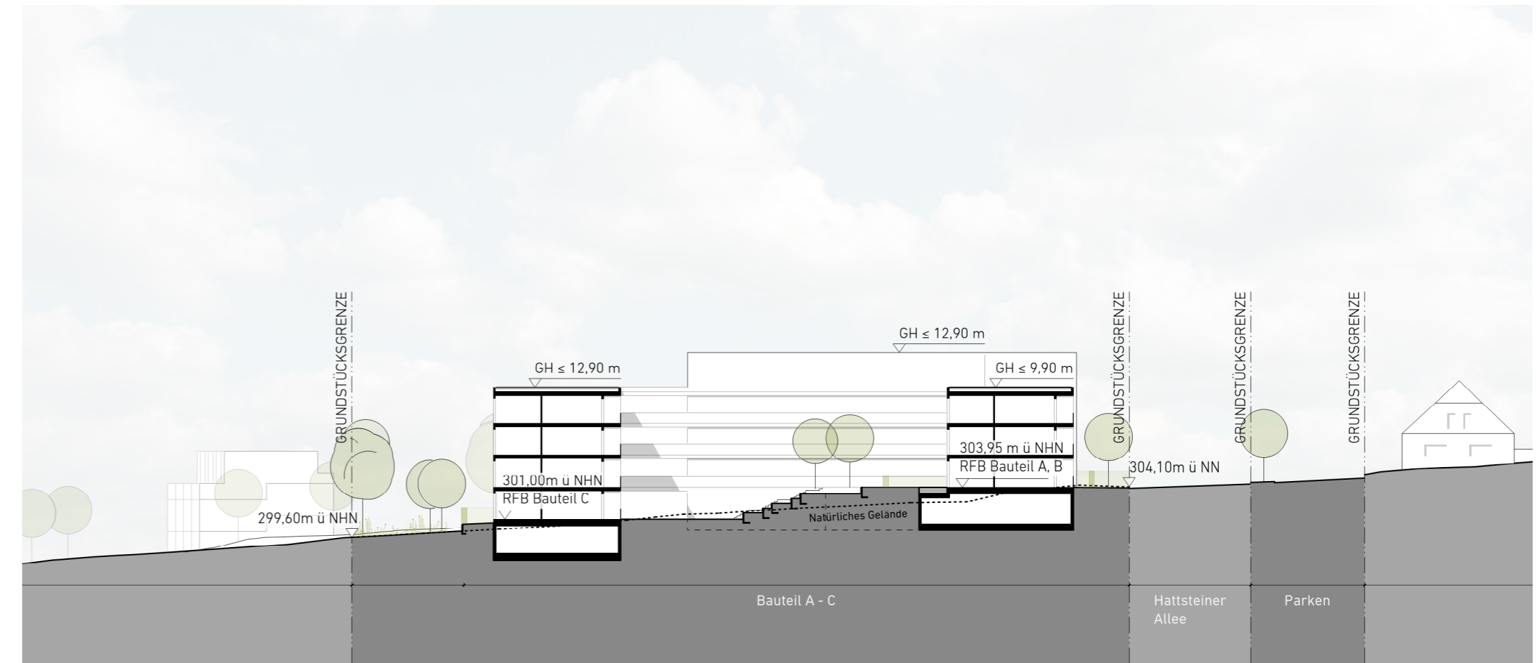
Schnitt B-B
