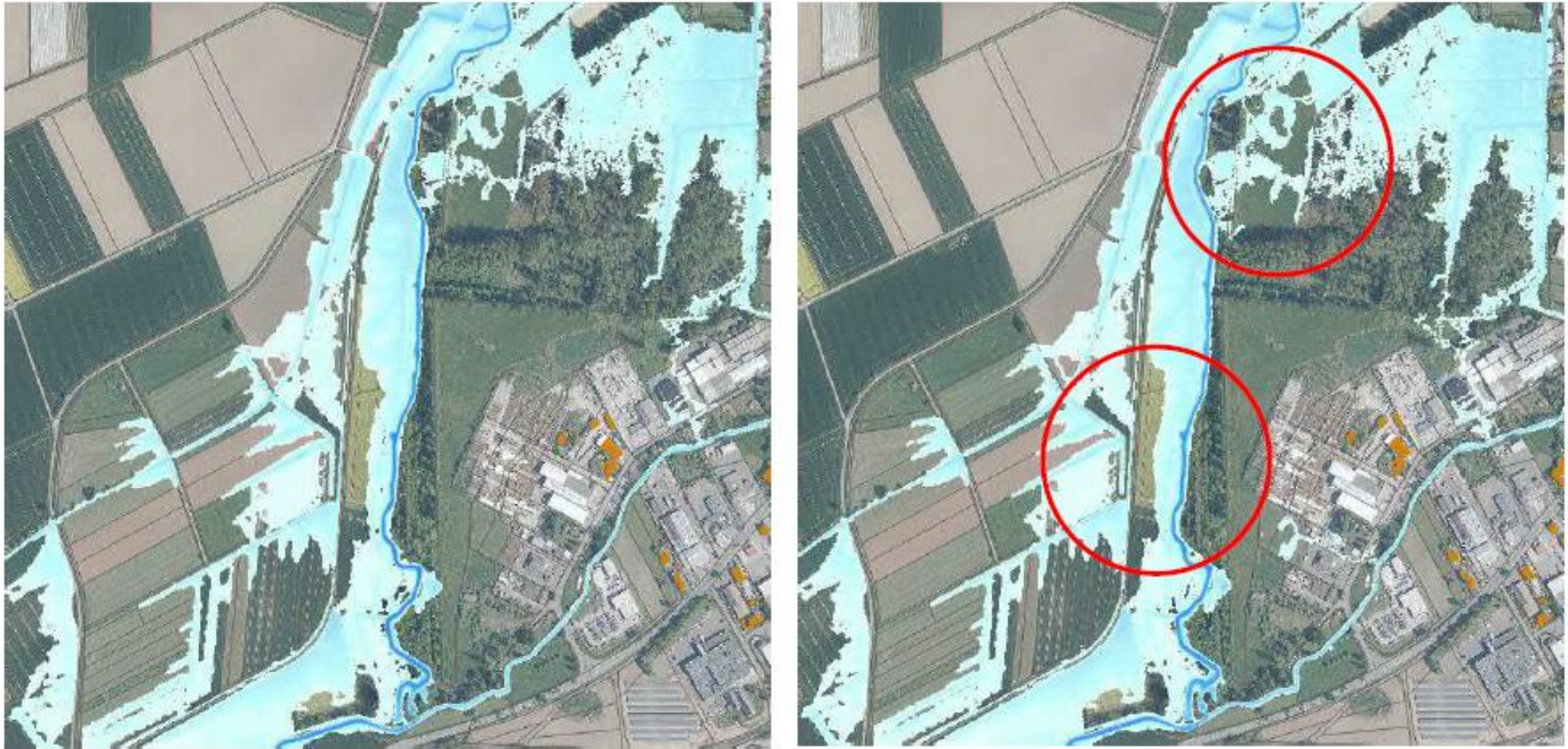
Abbildung 40: HQ 1 – Auswirkung der Variante b auf die Wassertiefen und das Überschwemmungsgebiet
