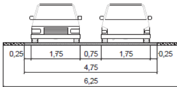
Bild 17: Begegnungsverkehr Pkw/Pkw auf zweistreifigem Verbindungsweg bei einer Geschwindigkeit von 50 km/h
