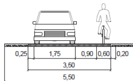
Bild 18: Begegnungsverkehr Pkw/Fahrrad auf einstreifigem Verbindungsweg bei sehr niedrigen Fahrgeschwindigkeiten
