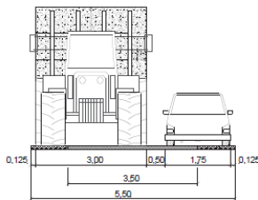
Bild 19: Begegnungsverkehr Traktor/ Pkw auf einstreifigem Verbindungsweg bei Schrittgeschwindigkeit
